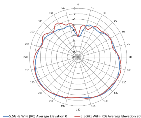
5.5GHz Wi-Fi天线方向图（垂直）
