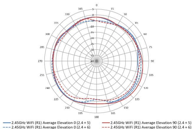
2.45GHz Wi-Fi天线方向图（垂直）
