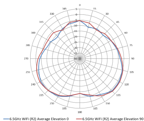
6.5GHz Wi-Fi天线方向图（垂直）
