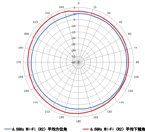
6.5GHz Wi-Fi天线方向图（水平）
