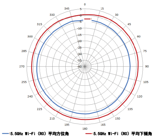
5.5GHz Wi-Fi天线方向图（水平）
