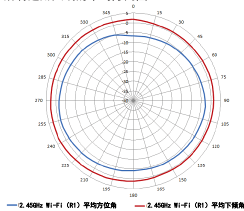
2.45GHz Wi-Fi天线方向图（水平）
